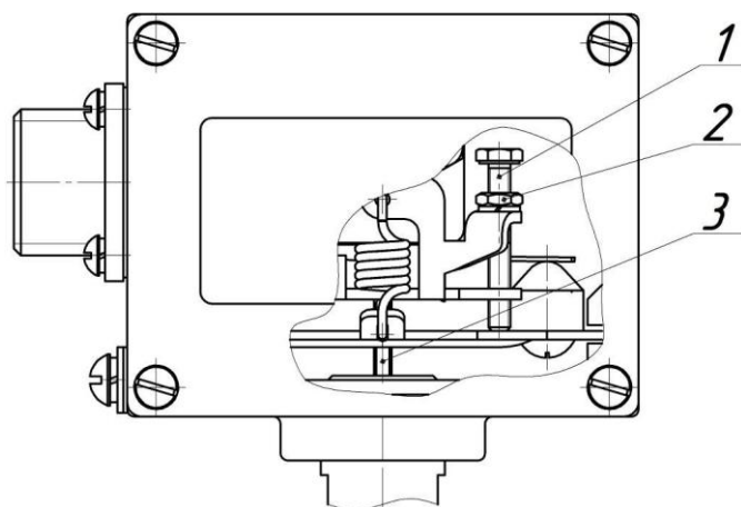
1 – винт настройки; 2 – гайка; 3 – шток
