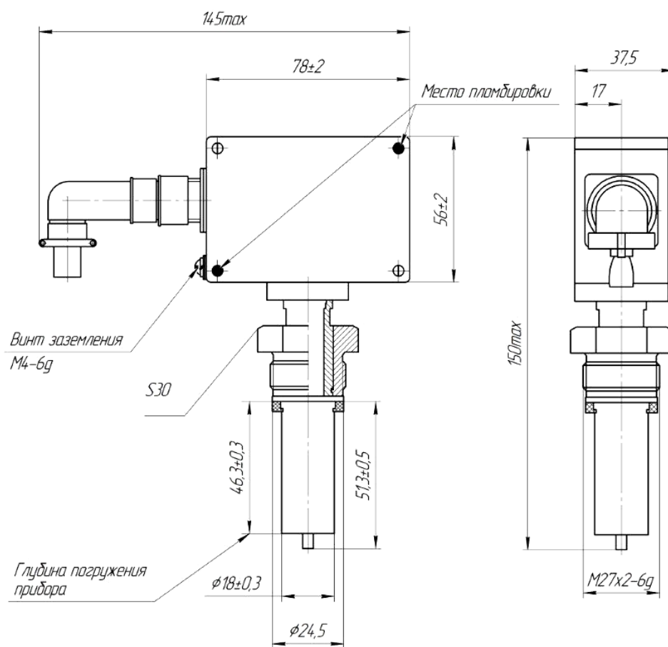
Рисунок А.1 – Датчик-реле температуры ТДМ-103 с соединителем типа 2РМДТ
