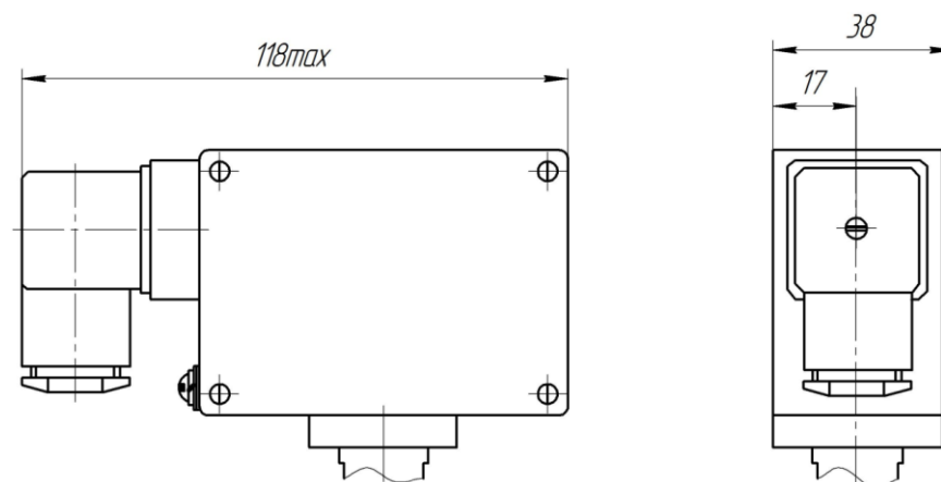
Рисунок А.2 – Датчик-реле температуры ТДМ-103 с соединителем по EN 175301-803 форма А
