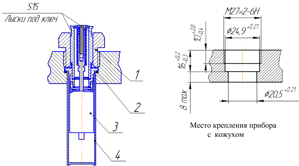
Рисунок А.3 – Крепление прибора без кожуха
